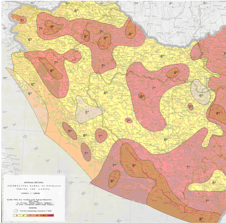
Intenzitet potresa za povratno razdoblje 200 godina
