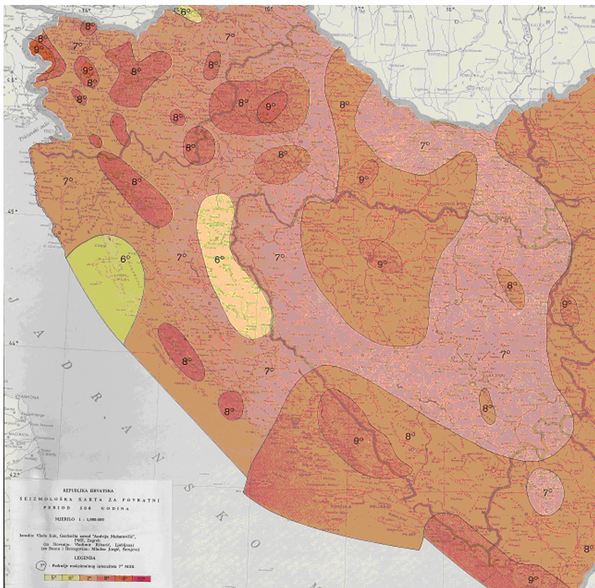
Intenzitet potresa za povratno razdoblje 500 godina
