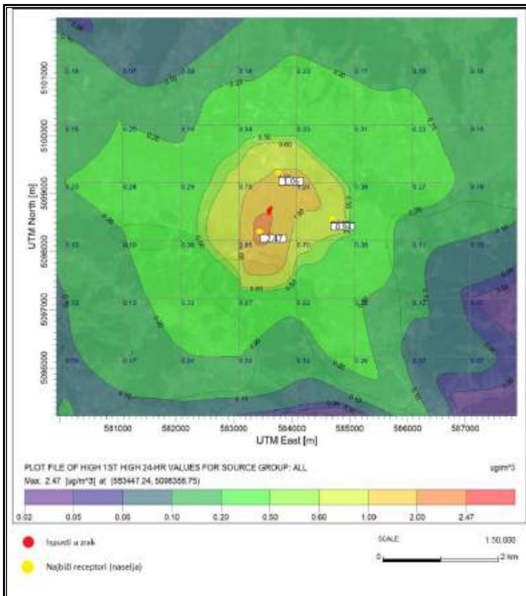
Slika 2.1 Model širenja onečišujuće tvari NH 3 za vrijeme usrednjavanja od 24 sata (Izvor: AERMOD View)
