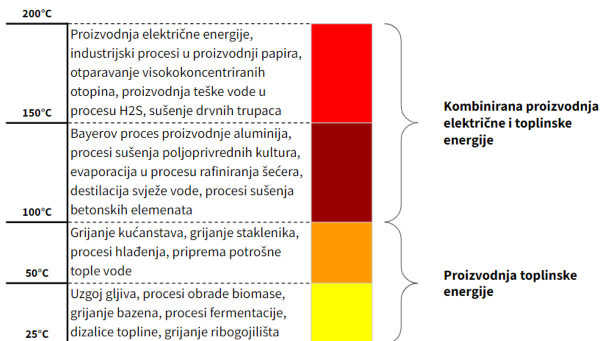
Slika 3: Mogućnosti primjene geotermalne energije razvrstane prema temperaturi geotermalnog fluida
