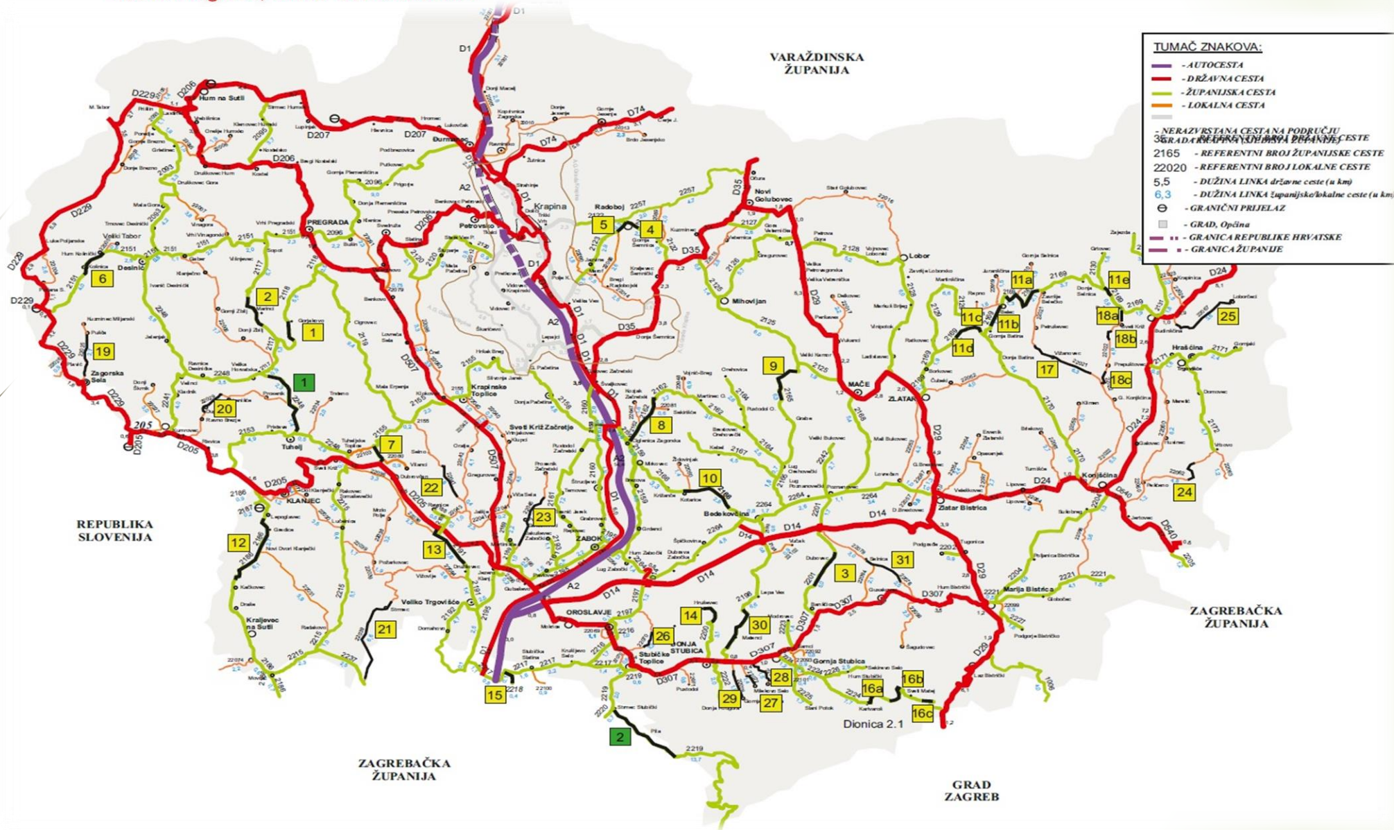
Karta 3. Interventna sanacija kolnika na dijelu županijskih i lokalnih cesta
